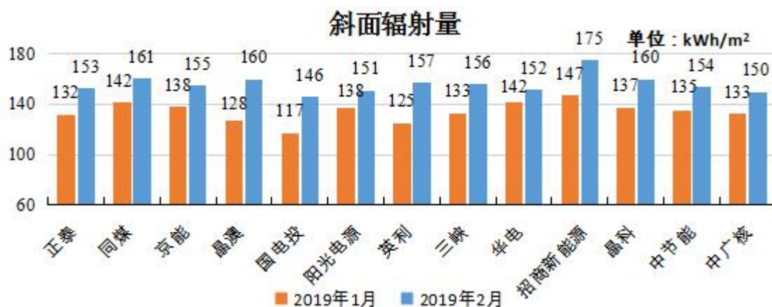
大同基地各项目斜面辐射量与环比变化
