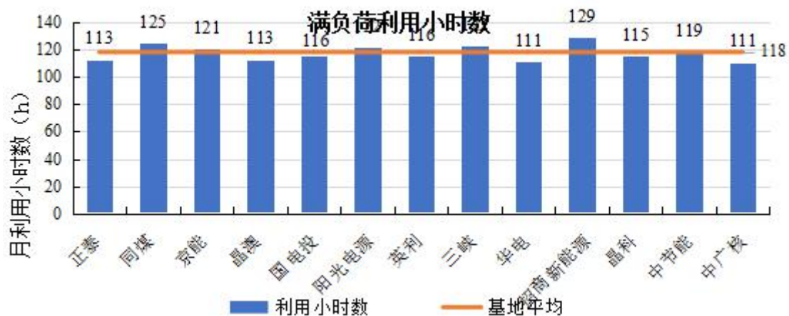
图 6 大同基地各项目满负荷利用小时数
